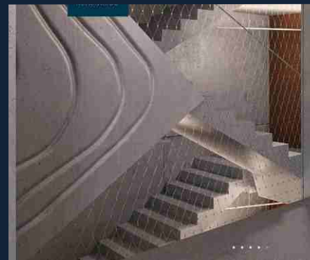
KOMUNARDŮ XXXV, PRAHA 8 (NEREZOVÉ SÍTĚ X-TEND® MW120/2,0) INTERIÉR, SCHODIŠTĚ, ZABRÁNĚNÍ PÁDU OSOB, ZÁBRADLÍ
