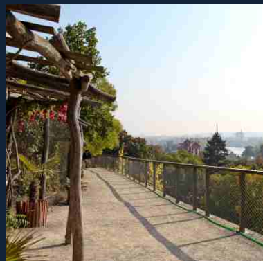
ZOO, PRAHA (NEREZOVÉ SÍTĚ X-TEND® MW40/1,5) EXTERIÉR, ZABRÁNĚNÍ PÁDU OSOB, ZÁBRADLÍ
